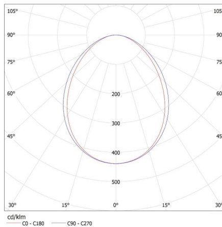
KANLUX S.A. (kat 33900) AL-SL-NW-MAT-W-NT / LDC (Polar)
