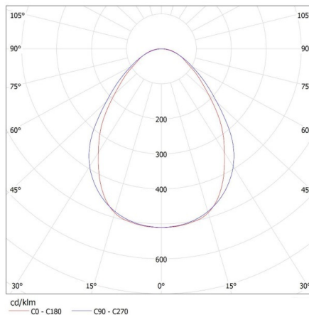
KANLUX S.A. (kat 33930) AL-SL-WW-MPR-S-NT / LDC (Polar)
