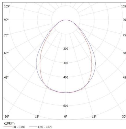
KANLUX S.A. (kat 33977) AL-MH-NW-MPR-W-NT / LDC (Polar)
