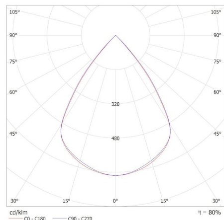
KANLUX S.A. (kat 33994) AL-ML-WW-RST-B-NT / Krzywa rozsyłu światła (biegunowo)
