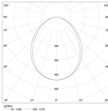
KANLUX S.A. (kat 34082) AL-LL-WW-MAT-W-NT / LDC (Polar)
