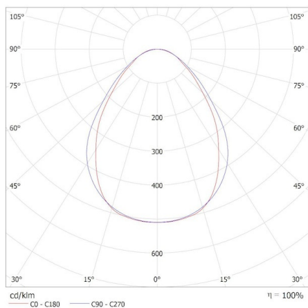
KANLUX S.A. (kat 35591) AL-MS-WW-MPR-W-NT / Krzywa rozsyłu światła (biegunowo)
