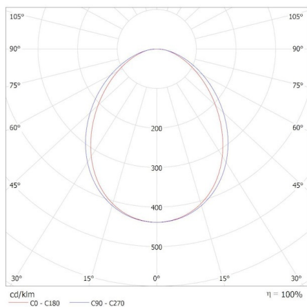
KANLUX S.A. (kat 35596) AL-MS-NW-MAT-S-NT / Krzywa rozsyłu światła (biegunowo)
