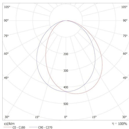
KANLUX S.A. (kat 35738) AL-LHAS-NW-MAT-W-NT / Krzywa rozsyłu światła (biegunowo)
