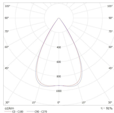
KANLUX S.A. (kat 35811) OS-S5D-WW-RST-W-N3 / Krzywa rozsyłu światła (biegunowo)
