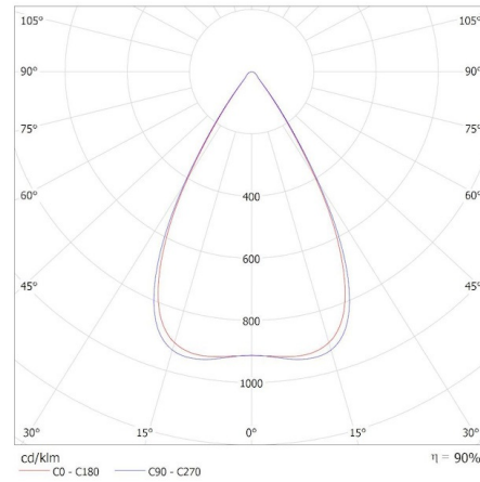
KANLUX S.A. (kat 35815) OS-L5D-WW-RST-W-N3 / Krzywa rozsyłu światła (biegunowo)
