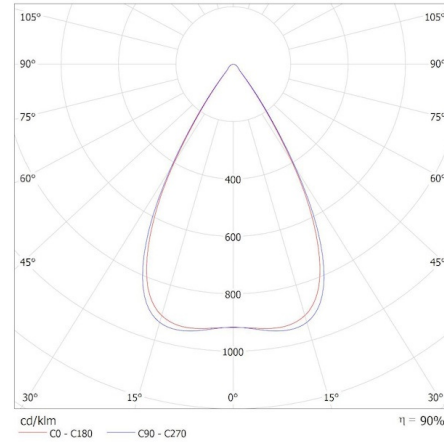
KANLUX S.A. (kat 35819) OS-M5D-WW-RST-W-N3 / Krzywa rozsyłu światła (biegunowo)
