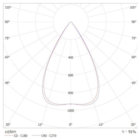
KANLUX S.A. (kat 35827) OS-S5D-NW-RST-W-N3 / Krzywa rozsyłu światła (biegunowo)
