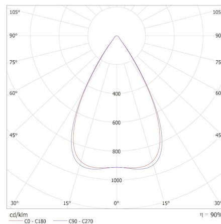
KANLUX S.A. (kat 35831) OS-L5D-NW-RST-W-N3 / Krzywa rozsyłu światła (biegunowo)
