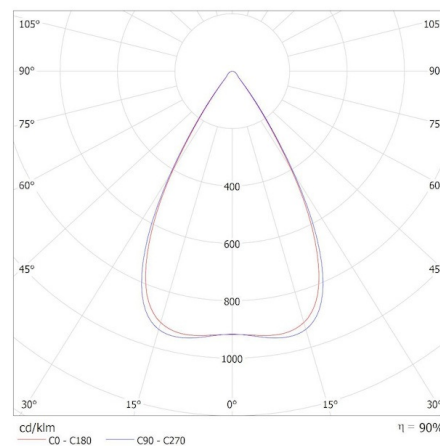
KANLUX S.A. (kat 35835) OS-M5D-NW-RST-W-N3 / Krzywa rozsyłu światła (biegunowo)
