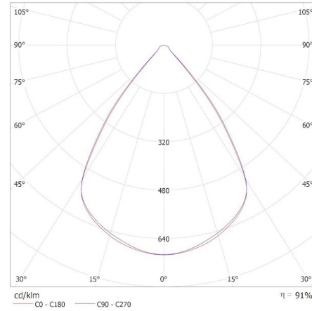
KANLUX S.A. (kat 35843) OS-S8D-WW-RST-W-N3 / Krzywa rozsyłu światła (biegunowo)
