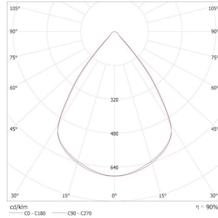
KANLUX S.A. (kat 35847) OS-L8D-WW-RST-W-N3 / Krzywa rozsyłu światła (biegunowo)
