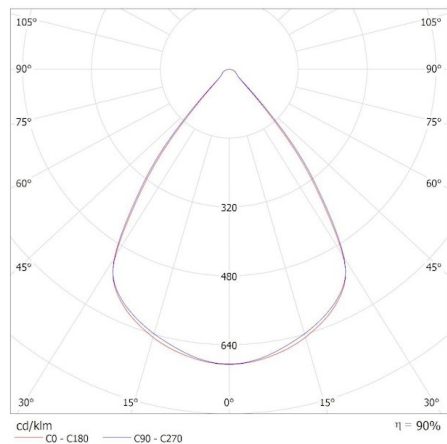
KANLUX S.A. (kat 35851) OS-M8D-WW-RST-W-N3 / Krzywa rozsyłu światła (biegunowo)
