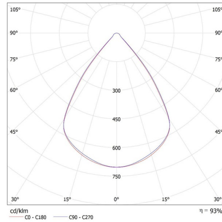
KANLUX S.A. (kat 35855) OS-H8D-WW-RST-W-N3 / Krzywa rozsytu światła (biegunowo)
