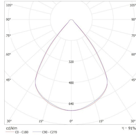
KANLUX S.A. (kat 35859) OS-S8D-NW-RST-W-N3 / Krzywa rozsyłu światła (biegunowo)
