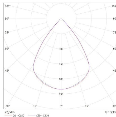
KANLUX S.A. (kat 35871) OS-H8D-NW-RST-W-N3 / Krzywa rozsyłu światła (biegunowo)
