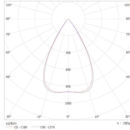
KANLUX S.A. (kat 35959) OS-L5D-NW-RST-B-N3 / Krzywa rozsyłu światła (biegunowo)
