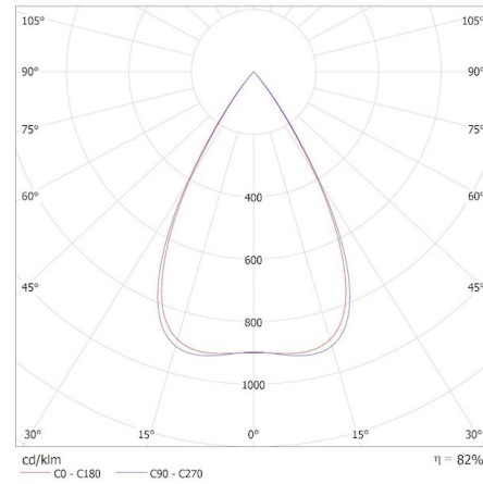
KANLUX S.A. (kat 35967) OS-H5D-NW-RST-B-N3 / Krzywa rozsyłu światła (biegunowo)
