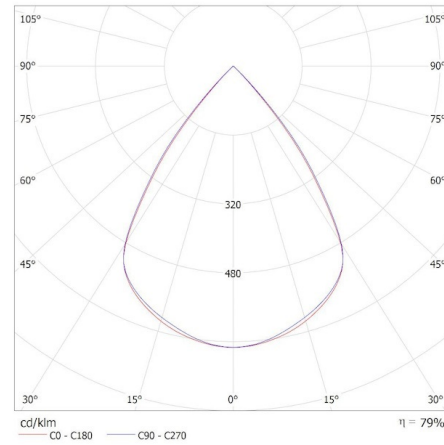
KANLUX S.A. (kat 35975) OS-L8D-WW-RST-B-N3 / Krzywa rozsyłu światła (biegunowo)
