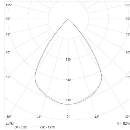
KANLUX S.A. (kat 35983) OS-H8D-WW-RST-B-N3 / Krzywa rozsyłu światła (biegunowo)
