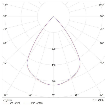
KANLUX S.A. (kat 35990) OS-L8D-NW-RST-B-N1 / Krzywa rozsyłu światła (biegunowo)
