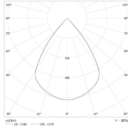
KANLUX S.A. (kat 35995) OS-M8D-NW-RST-B-N3 / Krzywa rozsyłu światła (biegunowo)
