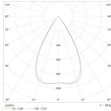
KANLUX S.A. (kat 36067) OS-S5D-WN-RST-W-N3 / Krzywa rozsyłu światła (biegunowo)
