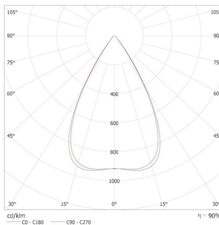
KANLUX S.A. (kat 36075) OS-M5D-WN-RST-W-N3 / Krzywa rozsyłu światła (biegunowo)
