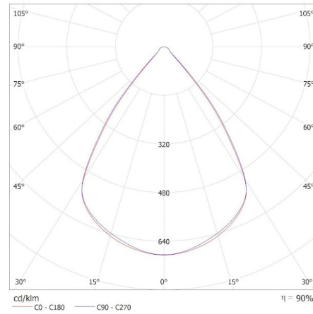
KANLUX S.A. (kat 36091) OS-M8D-WN-RST-W-N3 / Krzywa rozsyłu światła (biegunowo)
