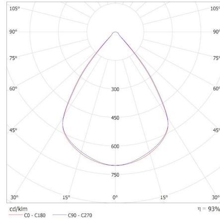
KANLUX S.A. (kat 36095) OS-H8D-WN-RST-W-N3 / Krzywa rozsyłu światła (biegunowo)
