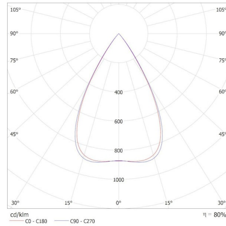
KANLUX S.A. (kat 36131) OS-S5D-WN-RST-B-N3 / Krzywa rozsyłu światła (biegunowo)
