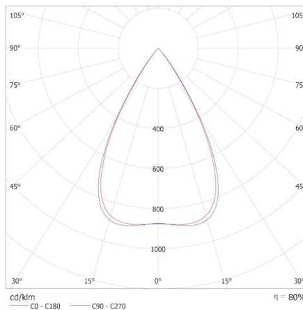
KANLUX S.A. (kat 36139) OS-M5D-WN-RST-B-N3 / Krzywa rozsyłu światła (biegunowo)
