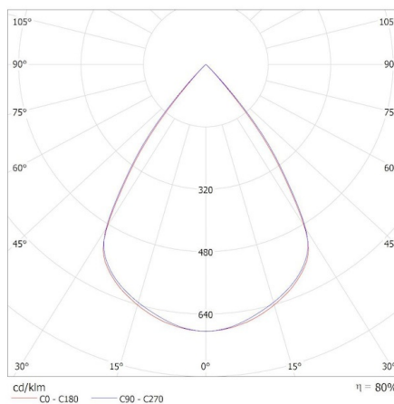
KANLUX S.A. (kat 36148) OS-S8D-WN-RST-B-P1 / Krzywa rozsyłu światła (biegunowo)
