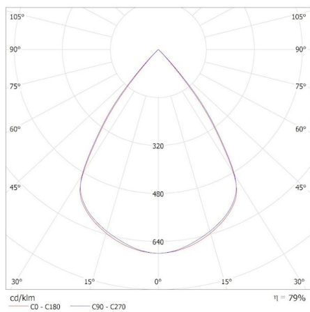
KANLUX S.A. (kat 36152) OS-L8D-WN-RST-B-P1 / Krzywa rozsyłu światła (biegunowo)
