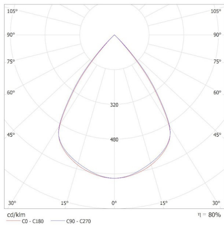
KANLUX S.A. (kat 36155) OS-M8D-WN-RST-B-N3 / Krzywa rozsyłu światła (biegunowo)
