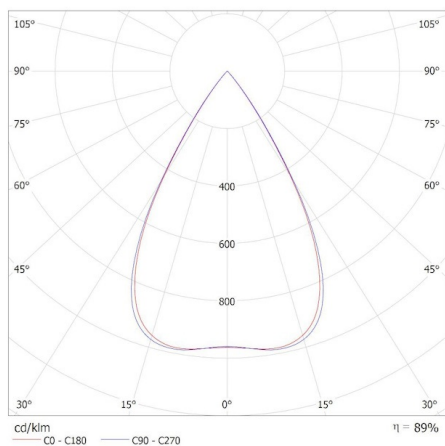
KANLUX S.A. (kat 36943) HR-MM-WW-W-NT / Krzywa rozsyłu światła (biegunowo)
