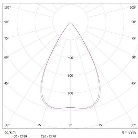
KANLUX S.A. (kat 37111) HR-MH-WW-W-RM / Krzywa rozsyłu światła (biegunowo)
