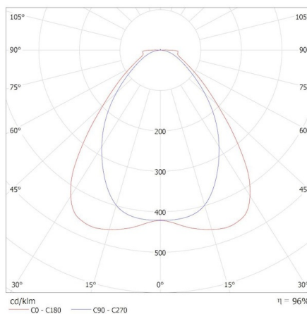
KANLUX S.A. (kat 37443) KN-S9D-WW-W-P1 / Krzywa rozsyłu światła (biegunowo)
