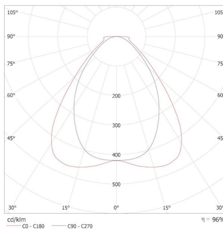
KANLUX S.A. (kat 37445) KN-M9D-WW-W-P1 / Krzywa rozsyłu światła (biegunowo)
