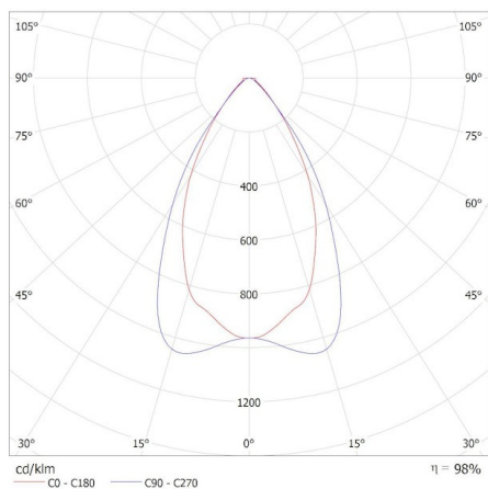
KANLUX S.A. (kat 37447) KN-L6D-NW-W-P1 / Krzywa rozsyłu światła (biegunowo)
