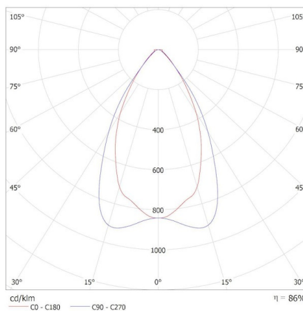
KANLUX S.A. (kat 37454) KN-M6D-WW-B-P1 / Krzywa rozsyłu światła (biegunowo)
