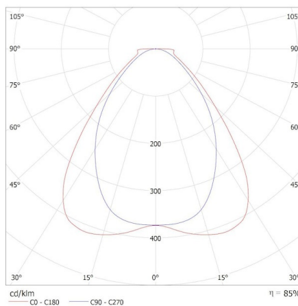
KANLUX S.A. (kat 37456) KN-L9D-WW-B-P1 / Krzywa rozsyłu światła (biegunowo)
