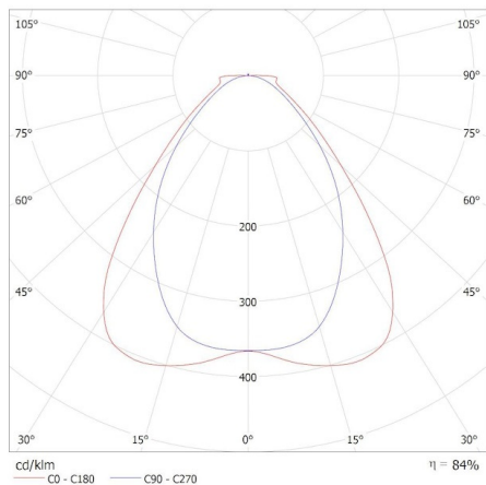
KANLUX S.A. (kat 37457) KN-M9D-WW-B-P1 / Krzywa rozsyłu światła (biegunowo)
