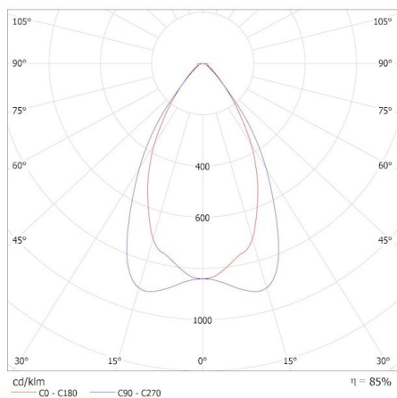
KANLUX S.A. (kat 37460) KN-M6D-NW-B-P1 / Krzywa rozsyłu światła (biegunowo)
