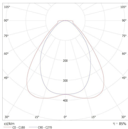
KANLUX S.A. (kat 37463) KN-M9D-NW-B-P1 / Krzywa rozsyłu światła (biegunowo)
