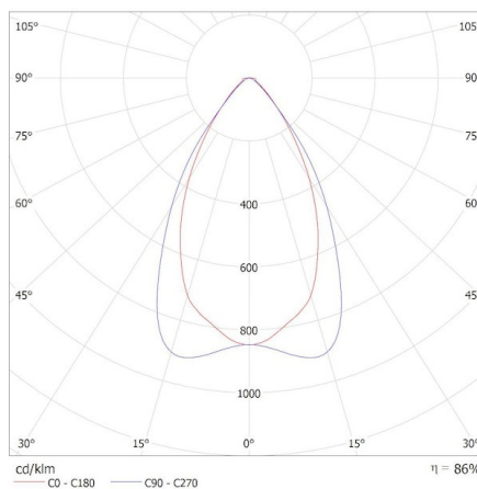
KANLUX S.A. (kat 37542) KNU-S6D-WW-B-P1D / Krzywa rozsyłu światła (biegunowo)
