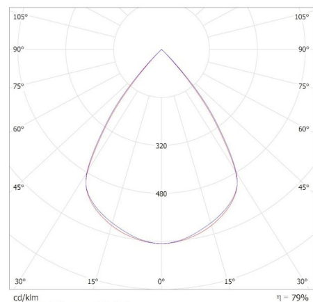
KANLUX S.A. (kat 38040) AL-MS-NW-RST-B-NT / Krzywa rozsyłu światła (biegunowo)
