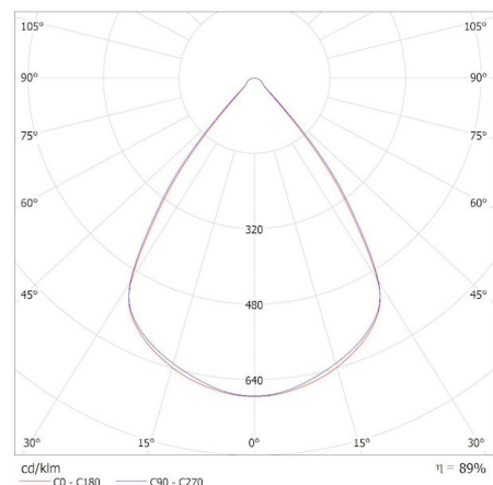
KANLUX S.A. (kat 38041) AL-MS-NW-RST-W-NT / Krzywa rozsyłu światła (biegunowo)
