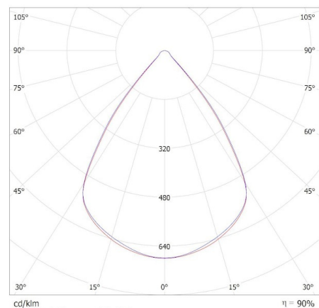
KANLUX S.A. (kat 38043) AL-MS-WW-RST-W-NT / Krzywa rozsyłu światła (biegunowo)
