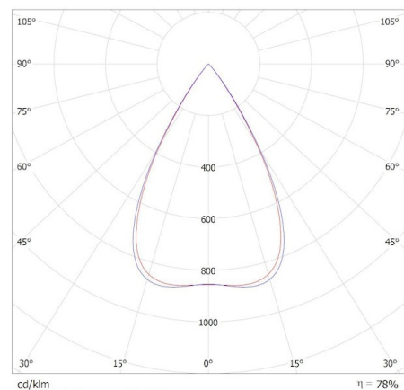
KANLUX S.A. (kat 38046) AL-MS5D-WW-RST-B-NT / Krzywa rozsyłu światła (biegunowo)
